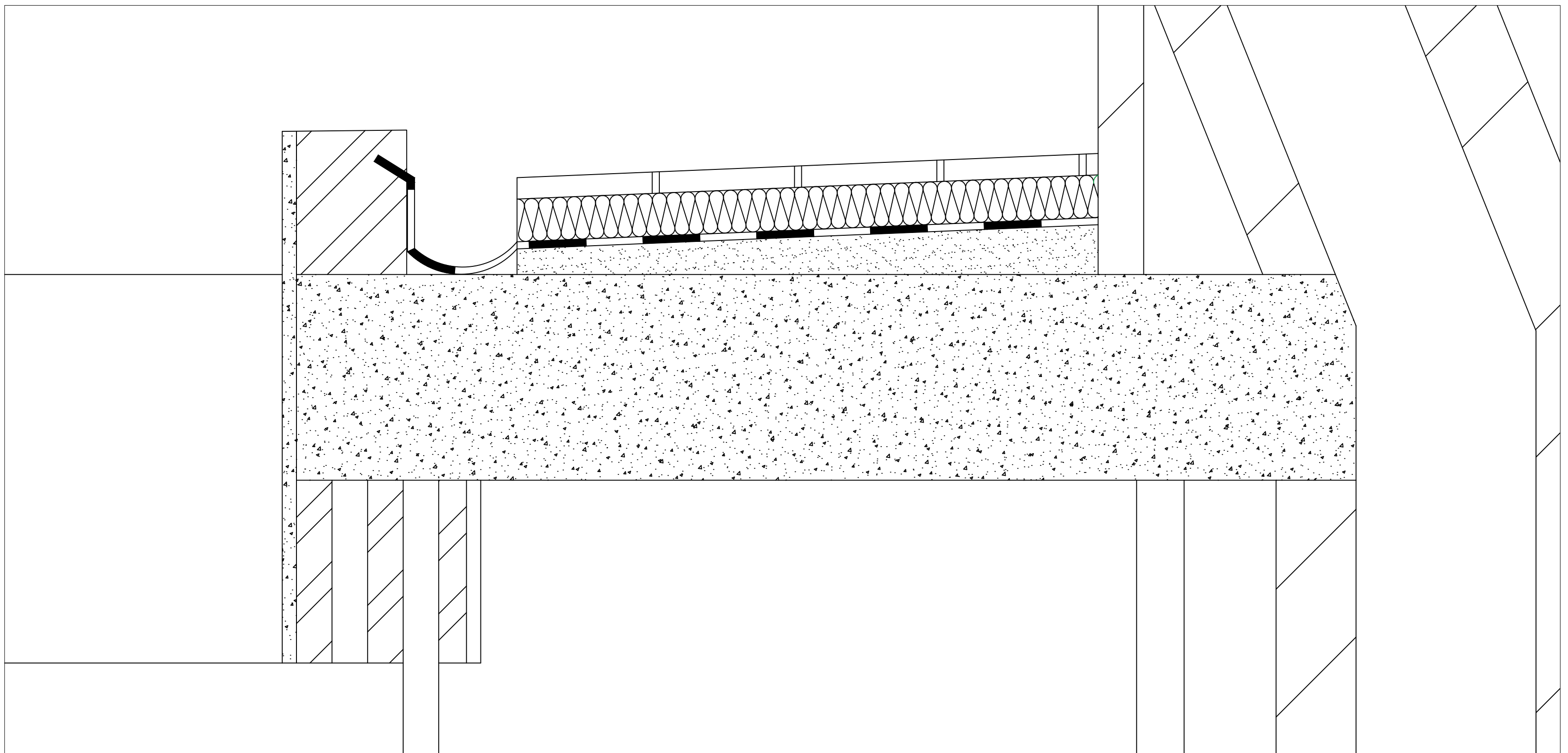
Pormenor cobertura 1:5
