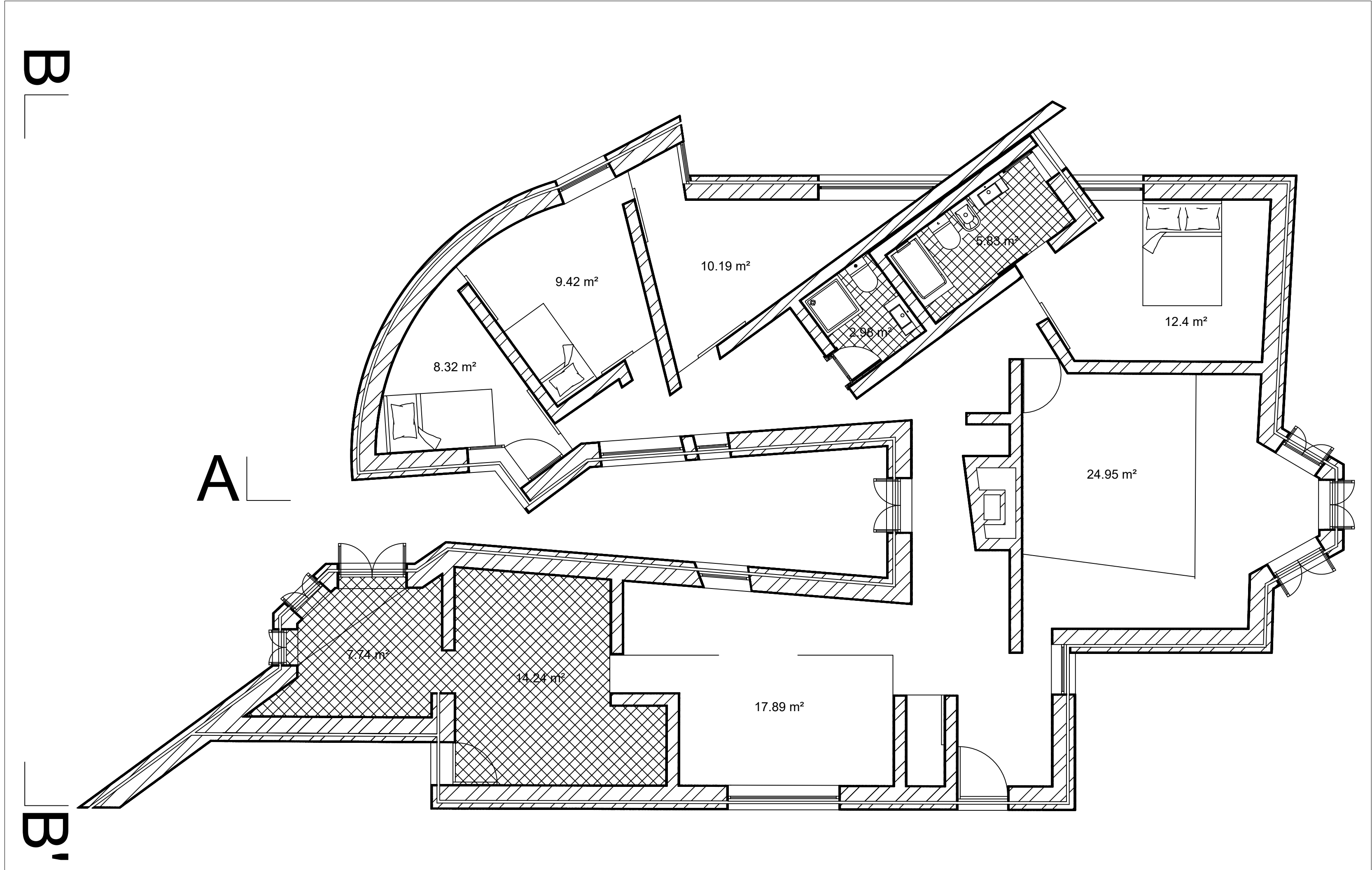
Planta 1:50
