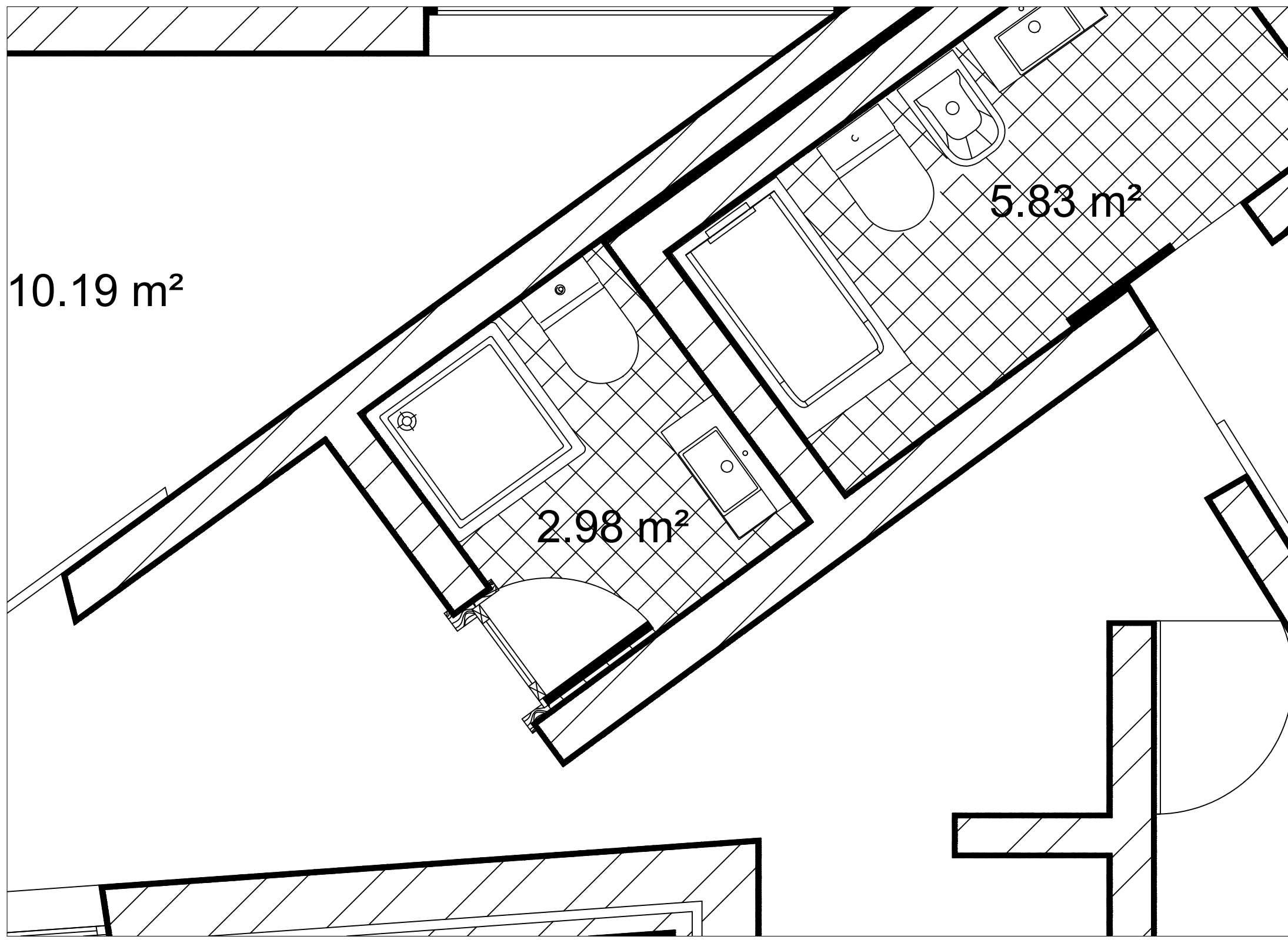
Extrato Planta 1:20
